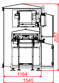
MEDIDAS DE CUCHILLA TSP-6
