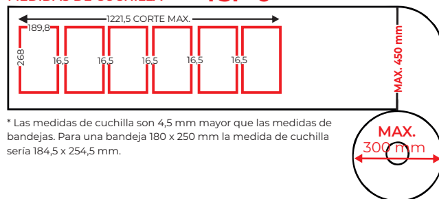
MEDIDAS DE CUCHILLA TSP-6
